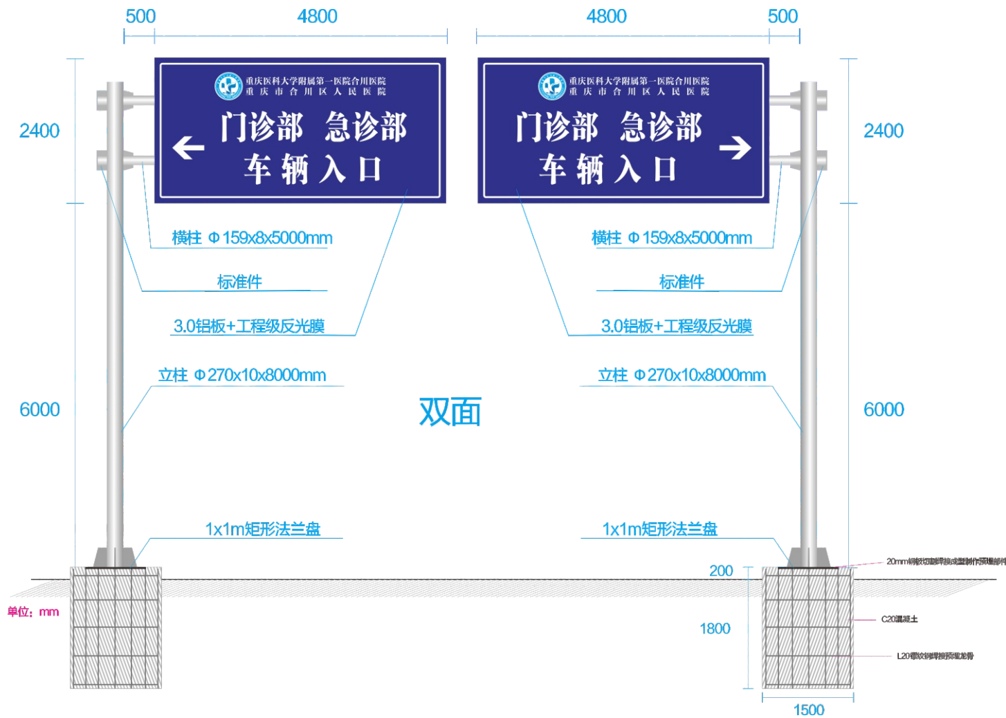
道路导视牌平面图一
