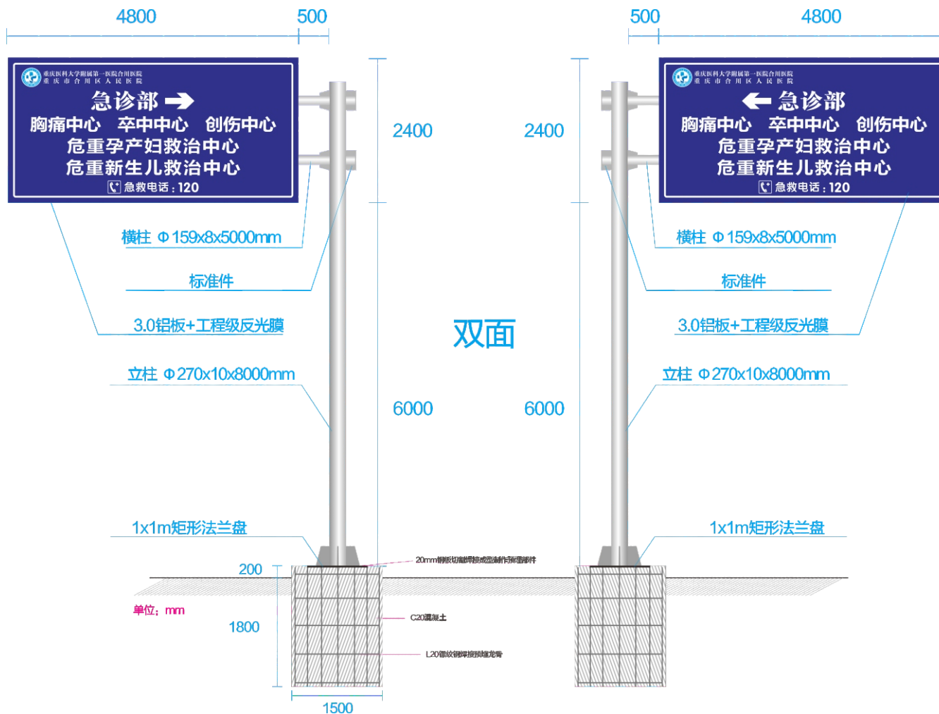
道路导视牌平面图三
